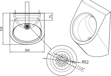
Detalle desagüe Válvula de Vacío/ Detail vacuum Valve
