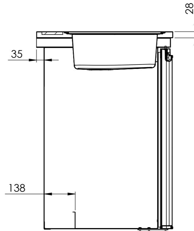
SECTION A-A
